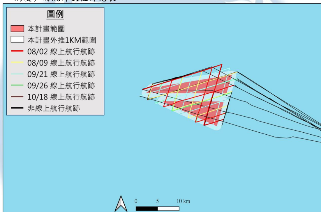
圖 2 2024 年颯妙風場位置及 9 條調查穿越線，每次出海調查隨機抽出三條進行調查，截至 113 年 10 月 31 日共 5 次調查。
